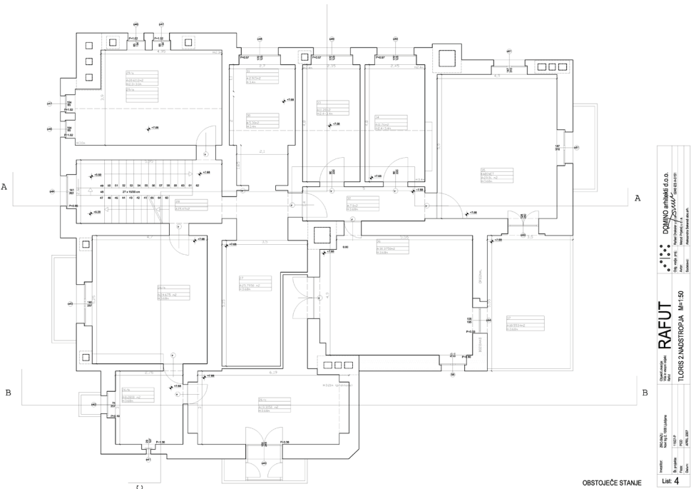
Tloris nadstropja
