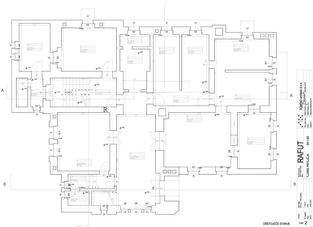
Tloris pritličja
