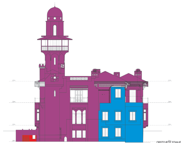
Zahodna fasada
