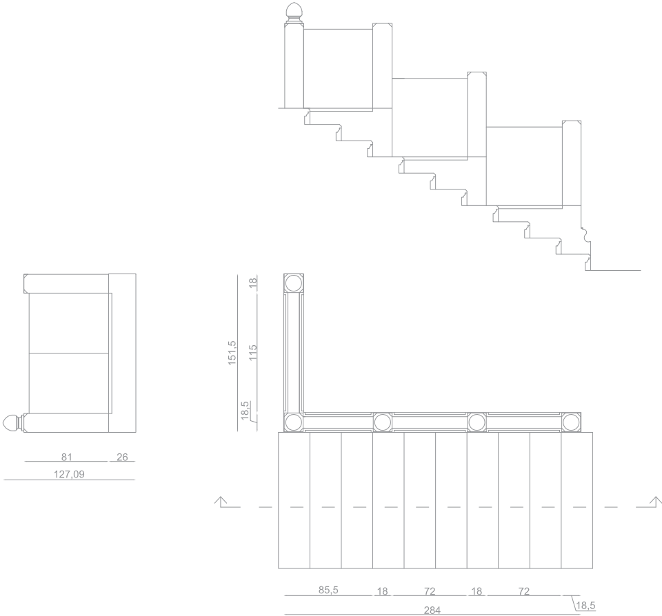
Kamnita ograja na notranjem glavnem stopnišču
