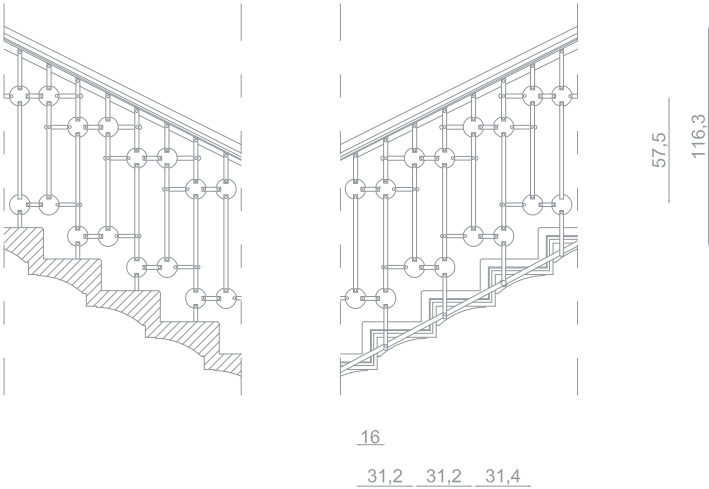
Kovana ograja na notranjem stranskem stopnišču
