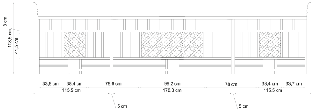
2 Ograja pri zaprti terasi z nadstreškom
