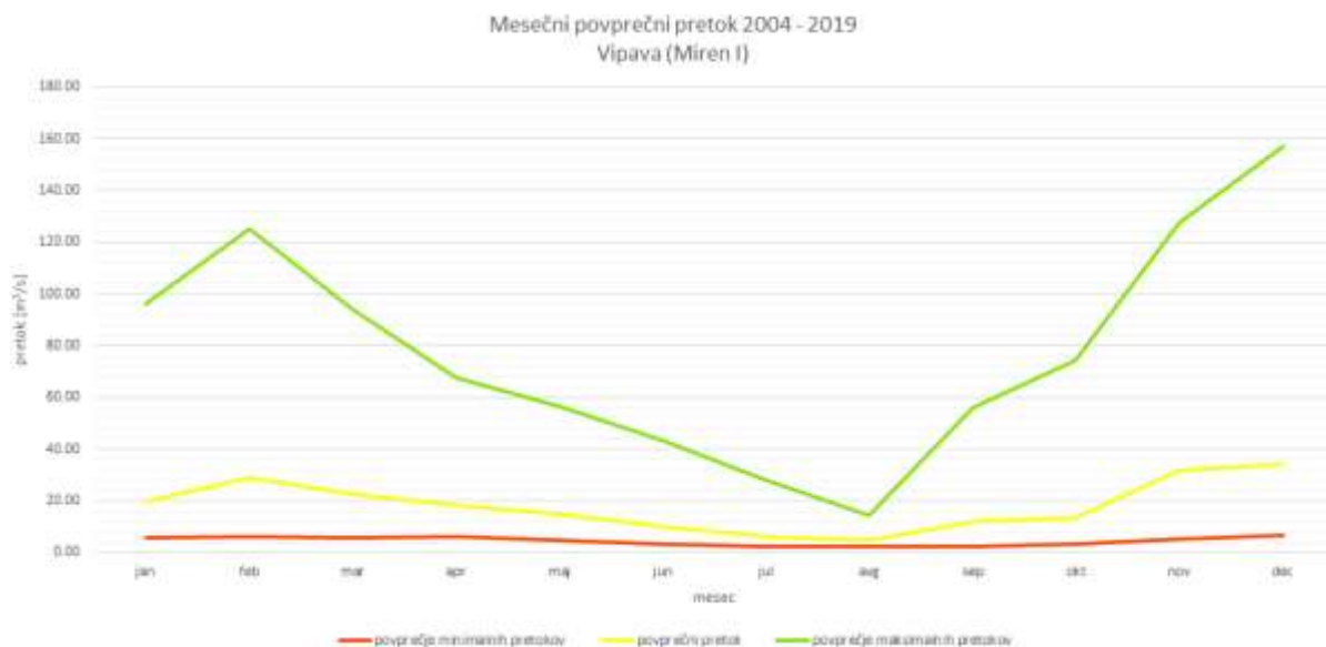
Slika 6.29: Povprečni minimalni, povprečni in povprečni maksimalni pretok reke Vipave na hidrogeološki postaji Miren I za obdobje 2004 - 2019.
