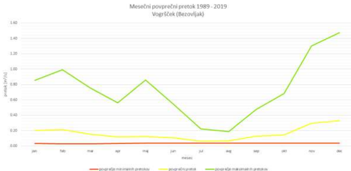
Slika 6.30: Povprečni minimalni, povprečni in povprečni maksimalni pretok potoka pod zajetjem Vogršček na hidrogeološki postaji Bezovljakl za obdobje 2004 - 2019.
