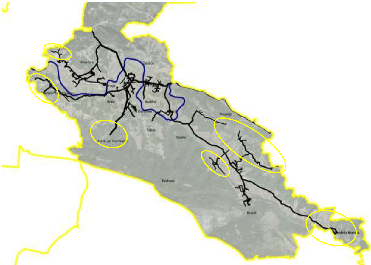
Slika 6.53: Prikaz identificiranih delov vodovodnega sistema na katerih je mogoče pričakovati težave s povišano temperaturo: Gradišče nad Prvačino, Potok pri Dornberku, Preseče, Brje, Pedrova, Spodnja Brana.
