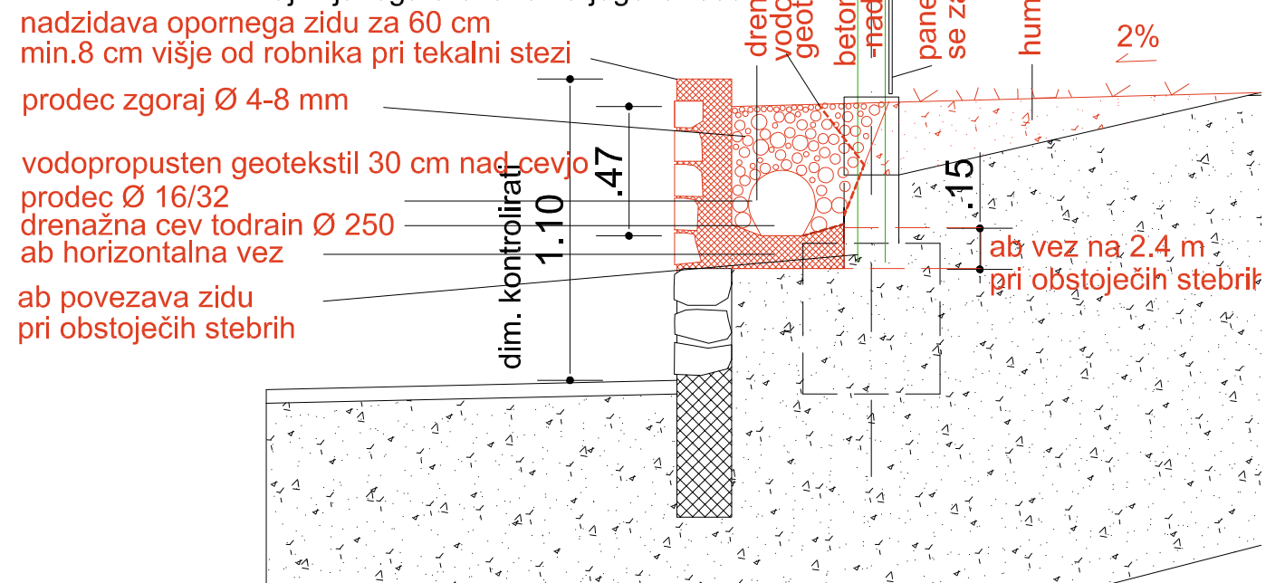
PREREZ B - B najnižja lega drenaže na jugozahodu
